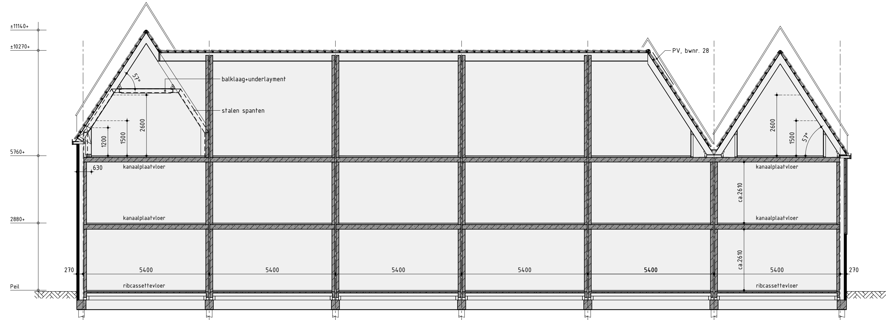
Principe doorsnede A-A
