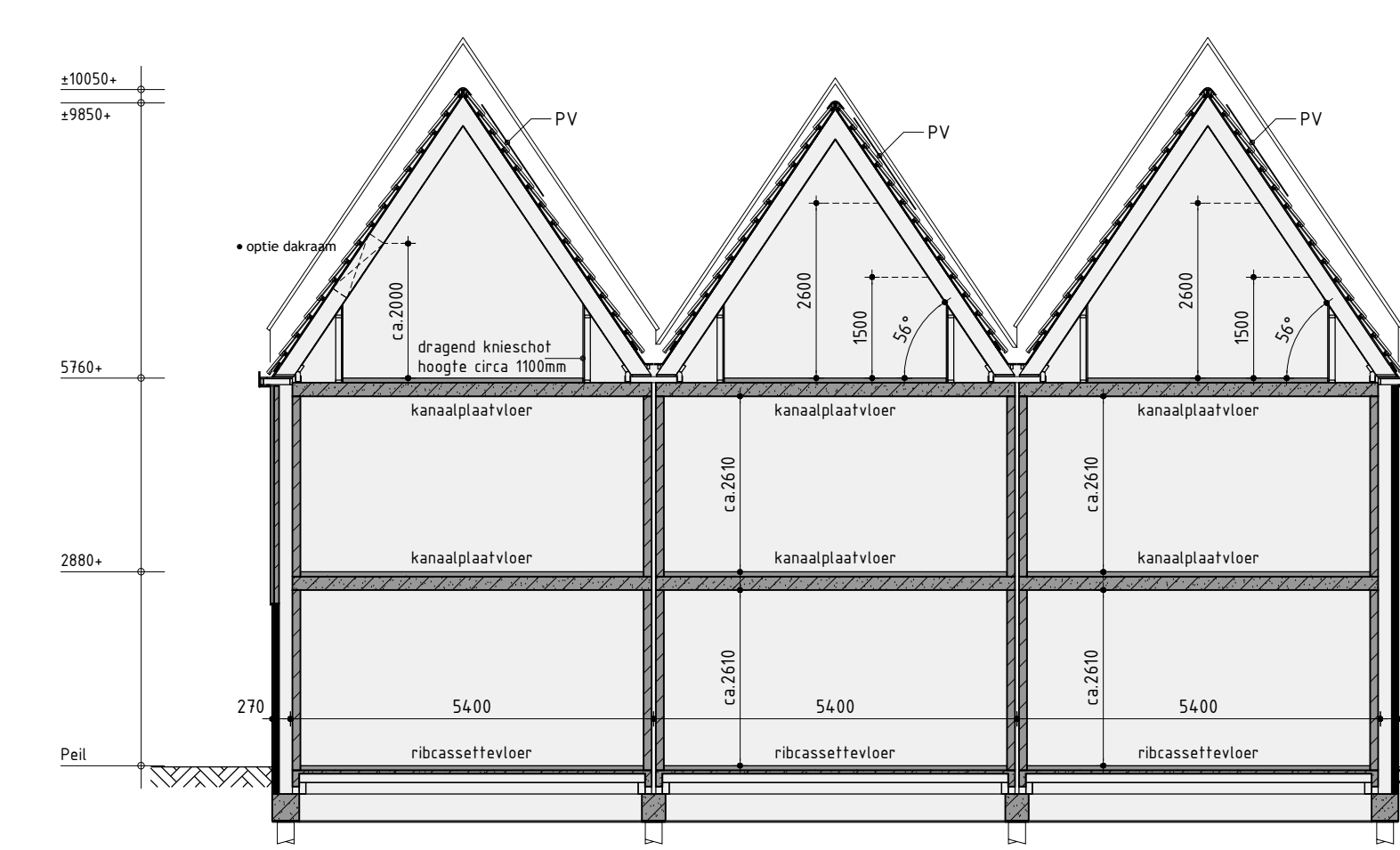
Principe doorsnede A-A
