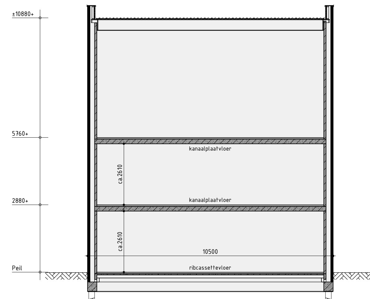
Principe doorsnede B-B
