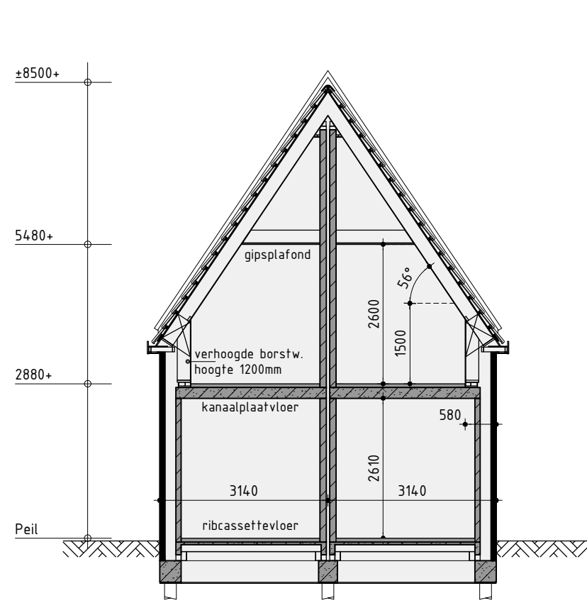
Principe doorsnede B-B
