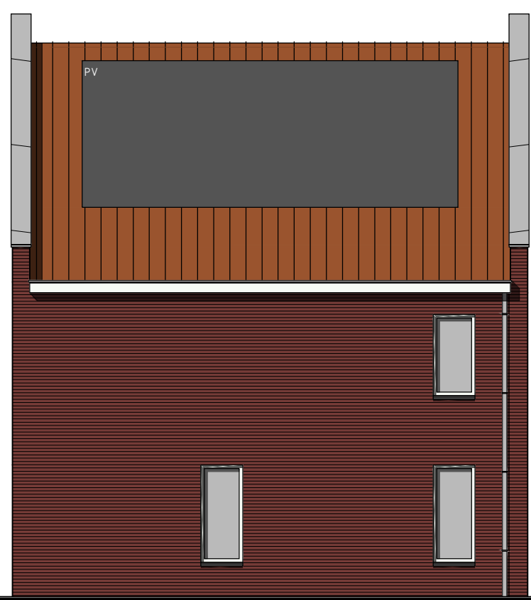
Rechter zijgevel
