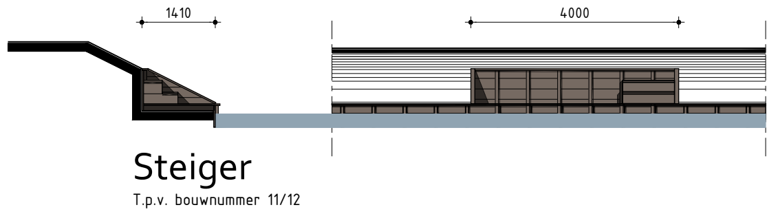
Principe doorsnede B-B
