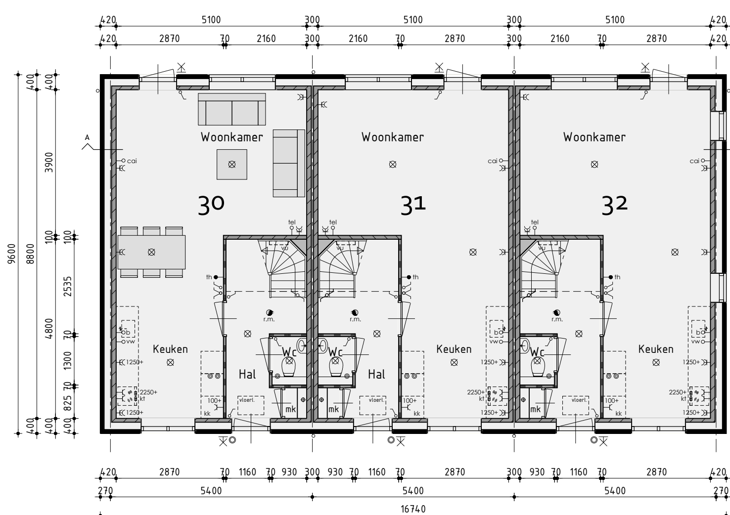
Begane grond v.z.v. vloerverwarming
