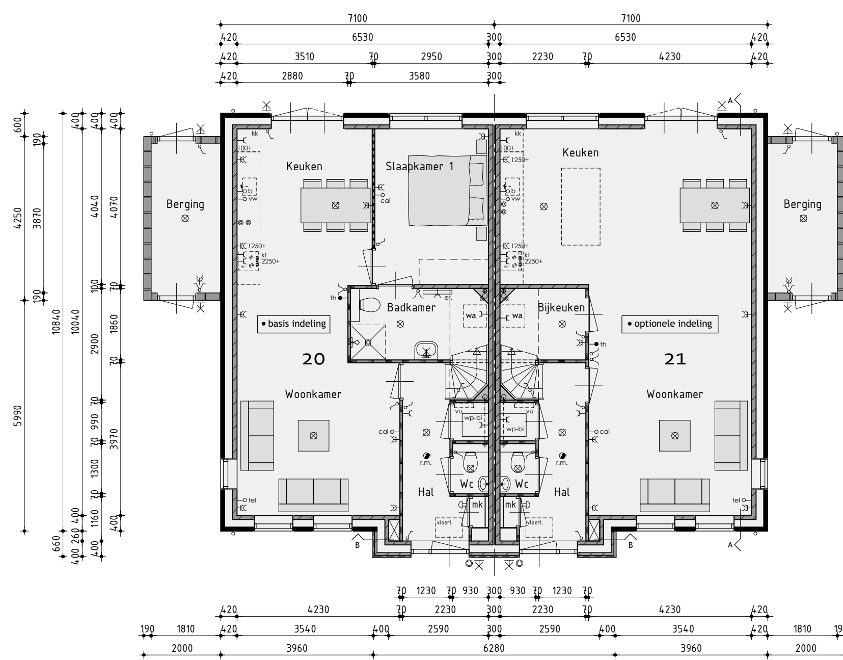
Begane grond v.z.v. vloerverwarming excl. berging
