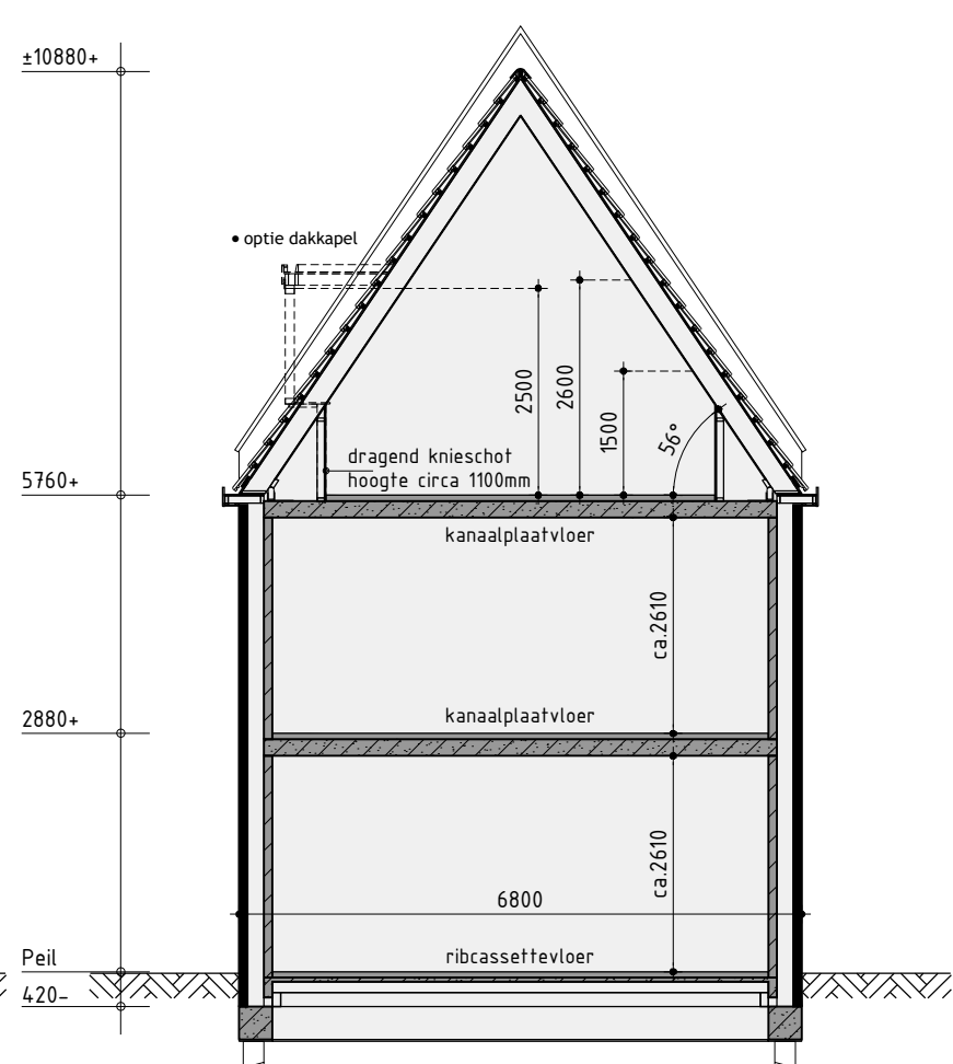
Principe doorsnede B-B
